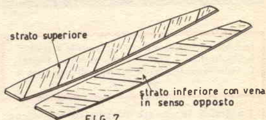
FIG. 7 FIANCATE REALIZZATE IN DOPPIO STRATO CON TAVOLETTE A VENA DIAGONALE
