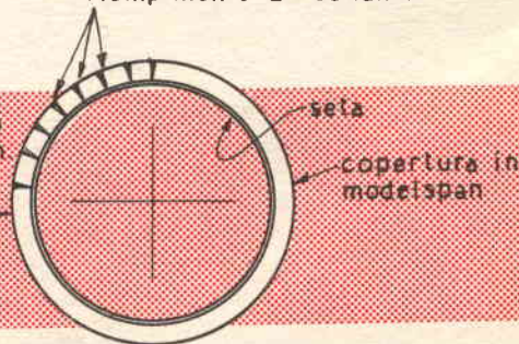
FIG.11 FUSOLIERA A TUBO CON TAVOLETTA INCISA
