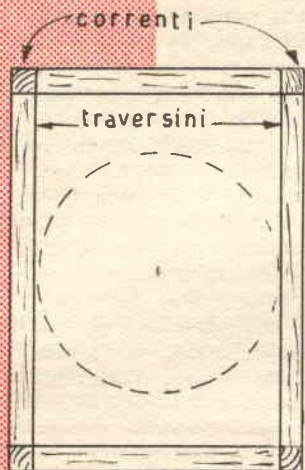
FIG. 1 - SEZIONE MINIMA DELLA FUSOLIERA
