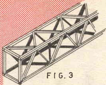
FIG. 3 COSTRUZIONE GEODETICA COMPLETA
