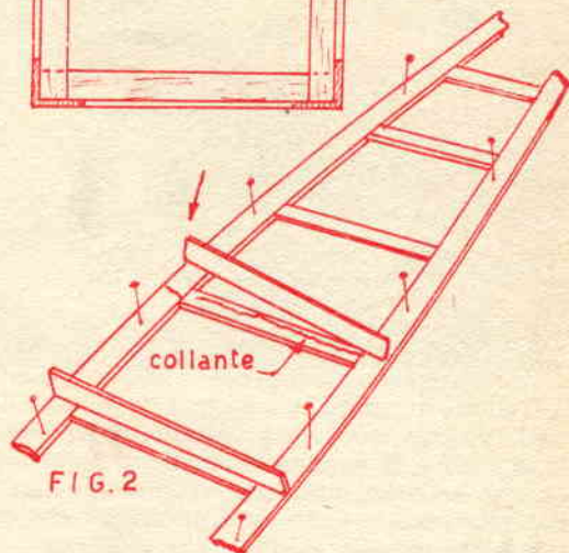
COSTRUZIONE CON CORRENTI AD L E TRAVERSINI A T.
